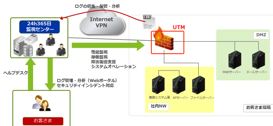
「SOMPO CYBER SECURITY UTM監視サービス」の利用イメージ
